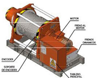
ISOMETRICO
