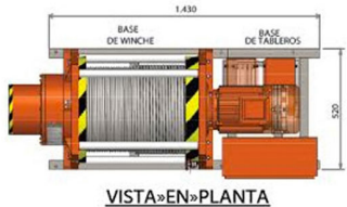
VISTA»EN»PLANTA
