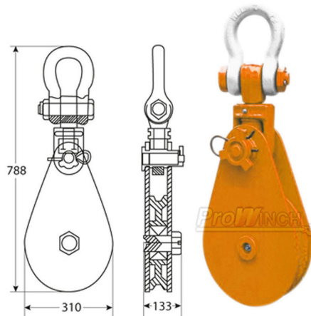
Dimensions in mm / Dimensiones en mm Imágenes Referenciales
