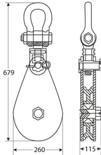
Dimensions in mm / Dimensiones en mm
