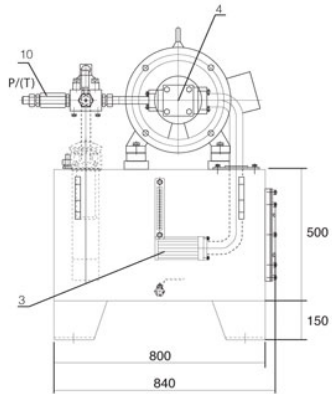
Dimensiones in mm / Dimensiones en mm
